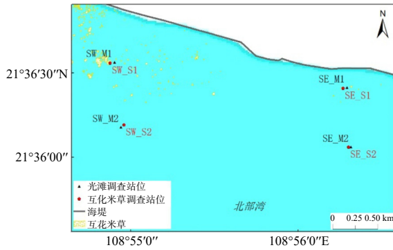
图 1 广西壮族自治区北部湾盐沼湿地采样站位
